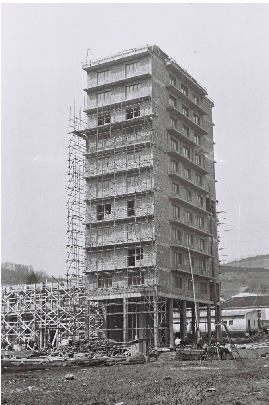
Слика 00. Објект Куле, североисточни изглед, током изградње (1960)
