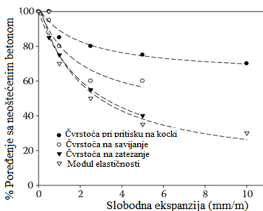
Слика 9. Слабење перформанси бетона услед АСР, [5]
