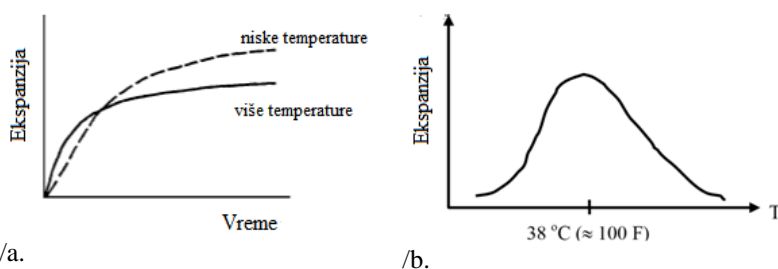
Слика 12/a. Криве експанзије бетона при нижим и вишим температурама, 12/b. Оптимална температура при којој је експанзија највећа, [4,5,12,16] и [19]
